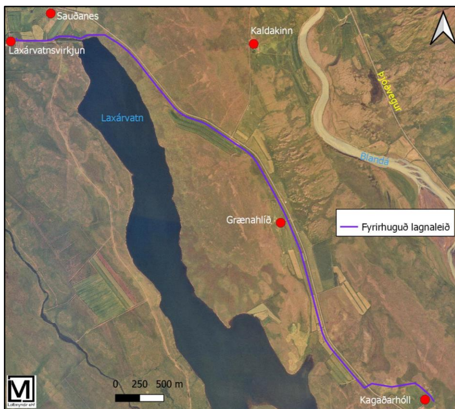
Mynd 3. Fyrirhuguð lagnaleið í utanverðum Langadal.
