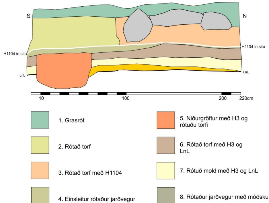
Mynd 5. Teikning sem sýnir mannvistarlög í vestursniði húsgrunns.
