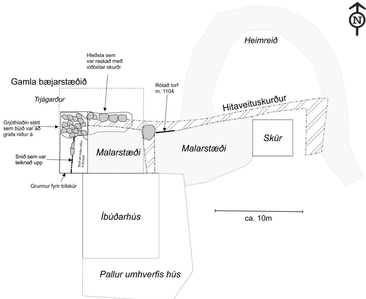
Mynd 2. Yfirlitstekning sem sýnir minjar í lagnaskurði og grunni að bílastæði á Sjöundastöðum. Myndin sýnir afstöðu minja en er ekki í nákvæmum skala.
