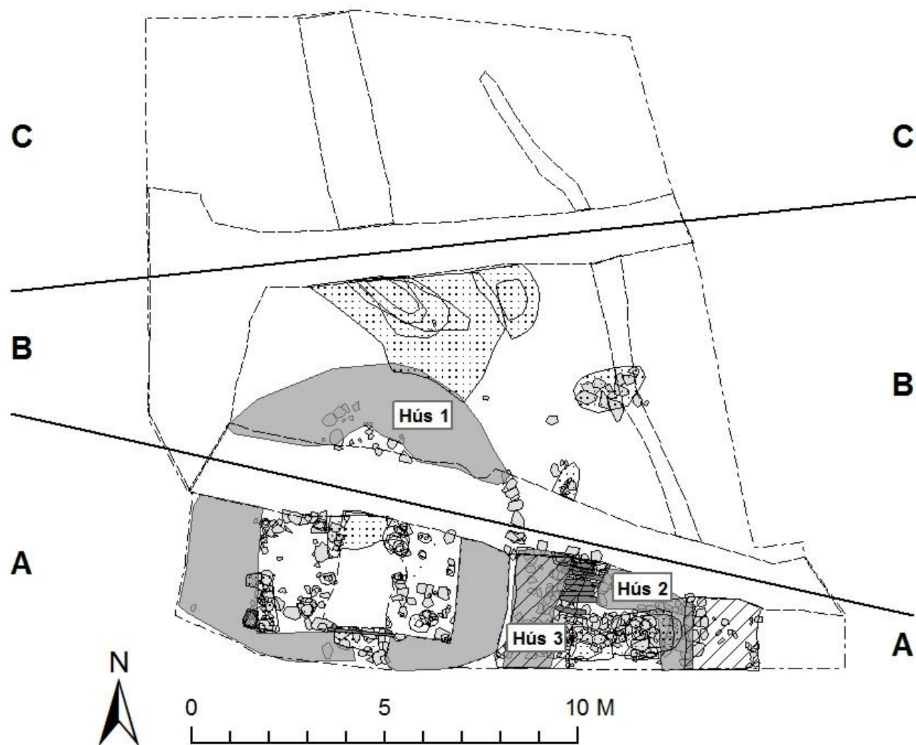
Yfirlitsmynd af byggingum og skiptingu uppgrftarins milli svæða
