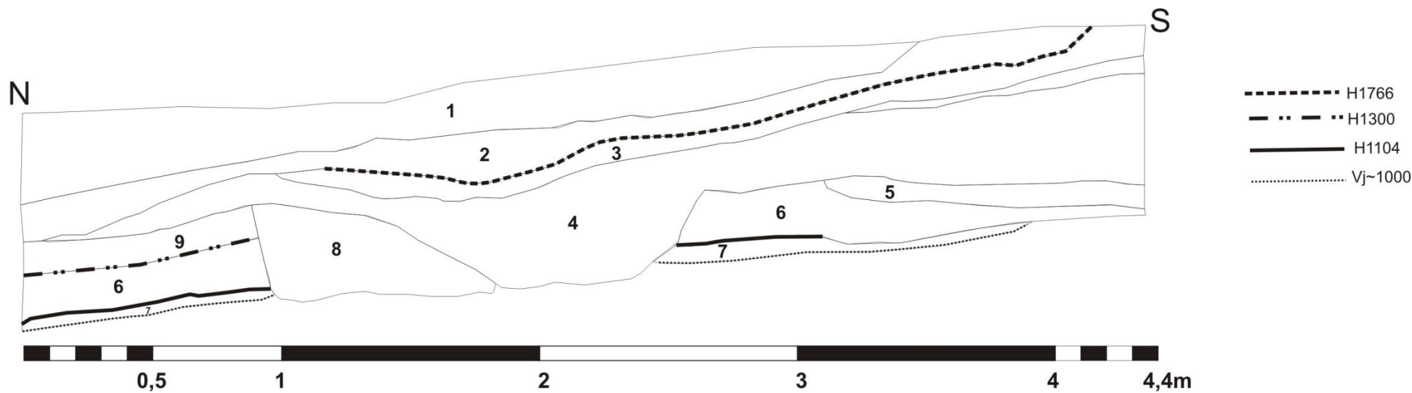
Snið 4 - austursnið í skurði sem snéri N-S á svæði C
