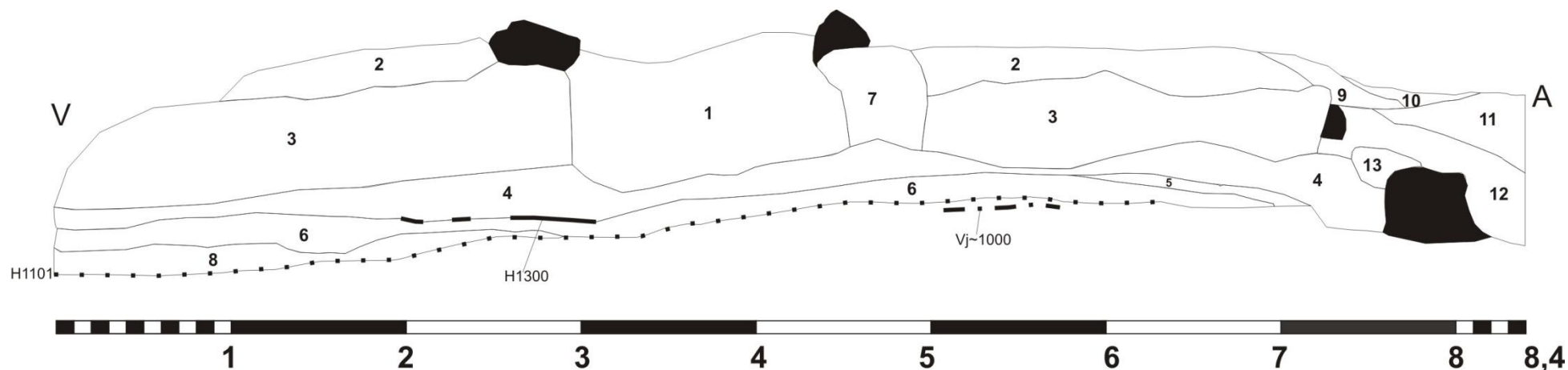
Snið 5 - norðursnið í svæði B (hluti sniðs 8 metrar af 11)
