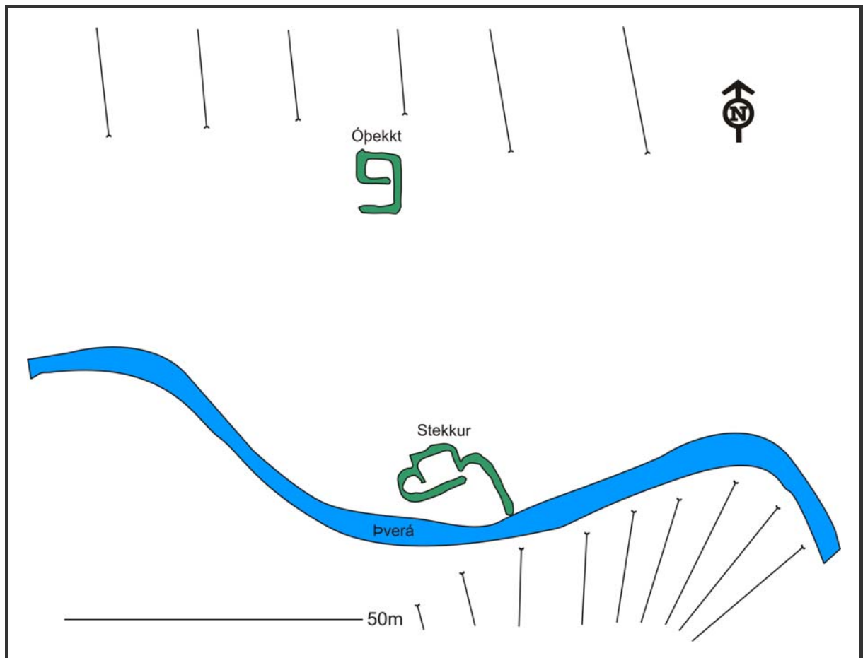
Teikning 7, Tóftir við Þverárgil. Frumteikning Hjalti Pálsson. Tölvuteikn. GSS.
