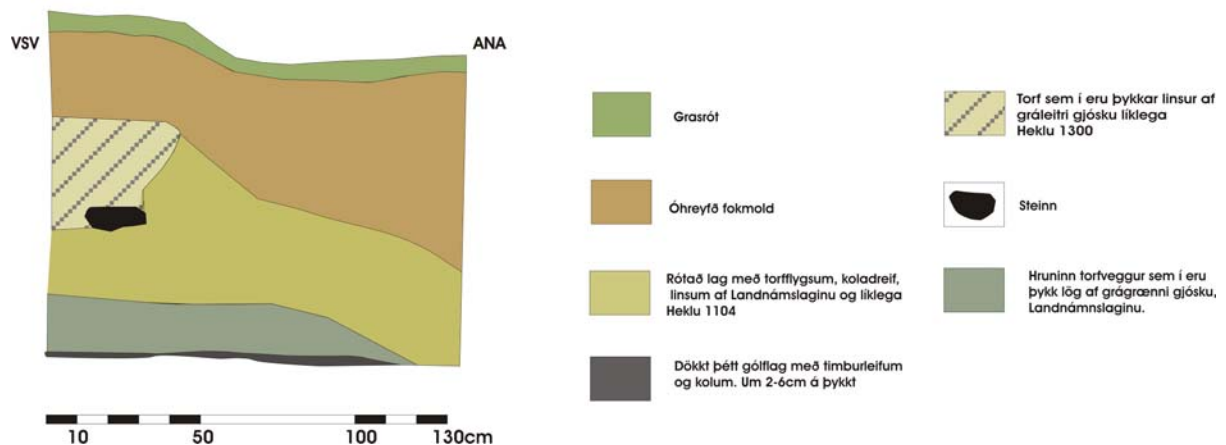
Mynd 15. Norðursnið í tóftavegg í Fögruhlíð.
