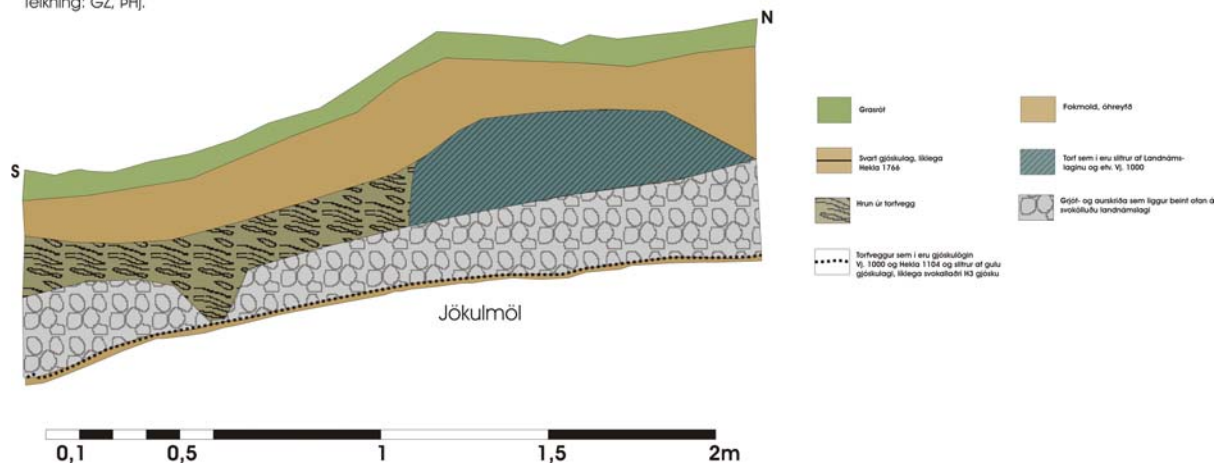
Mynd 23. Vestursnið í tóftarvegg, Grund, Öxnadalshéiði.
