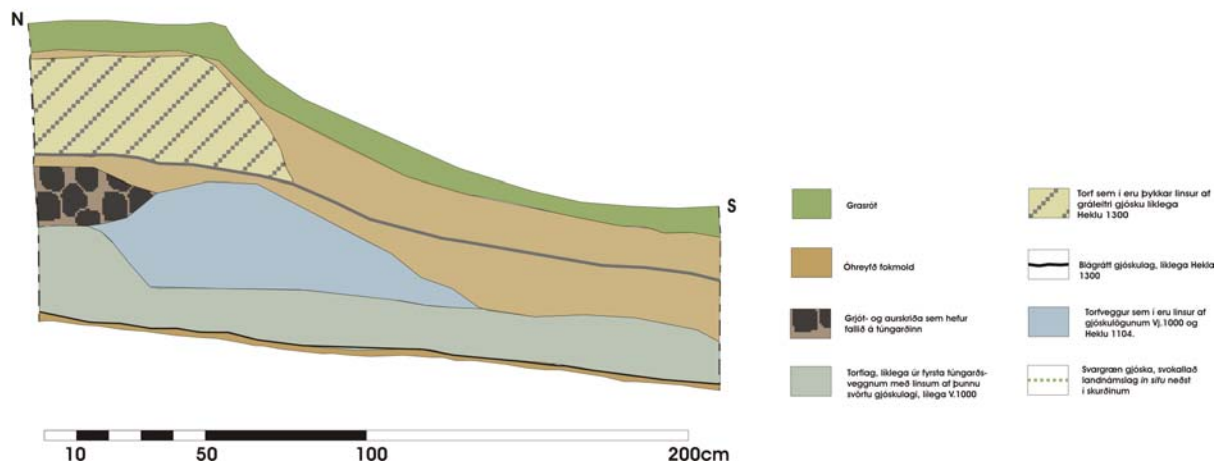
Mynd 11. Austurnið í túngarð á Ófriðarstöðum, Austurdal.
