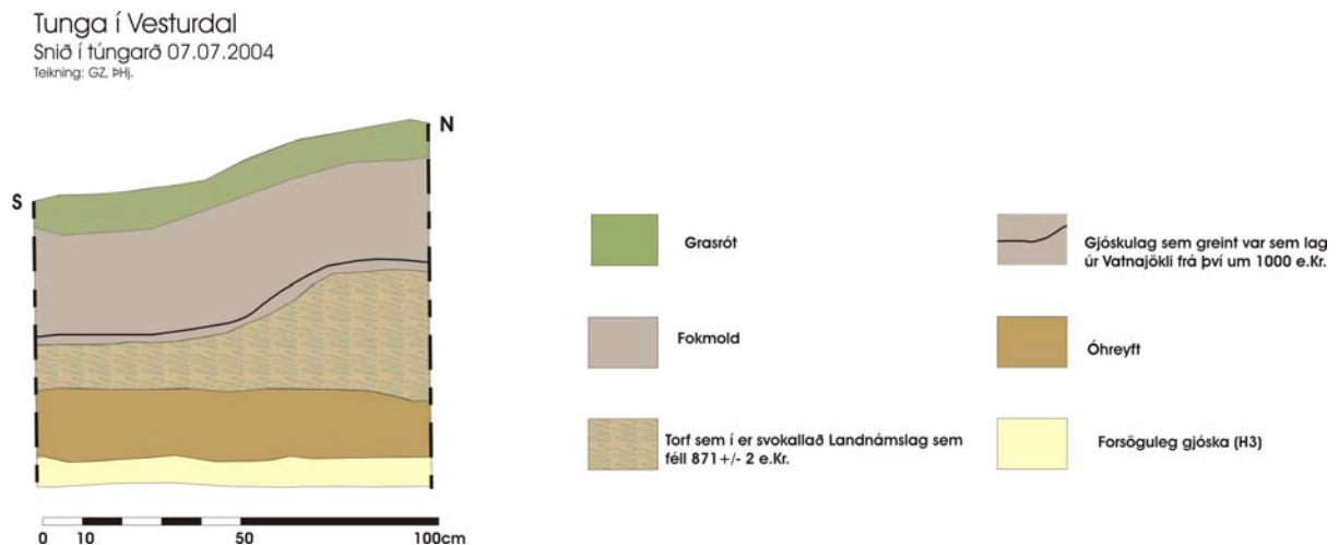
Mynd 3. Vestursnið í vallargarð í Tungu, Vesturdal.
