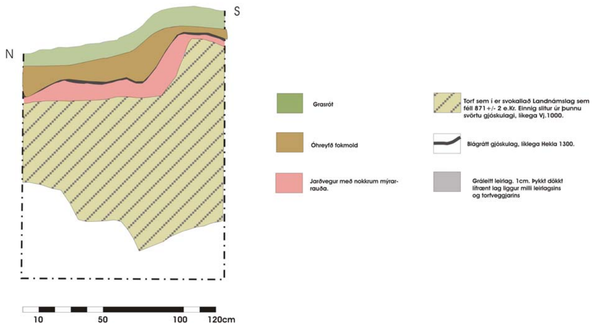
Mynd 4. Austursnið í tóftarvegg á Fossum, Vesturdal.
