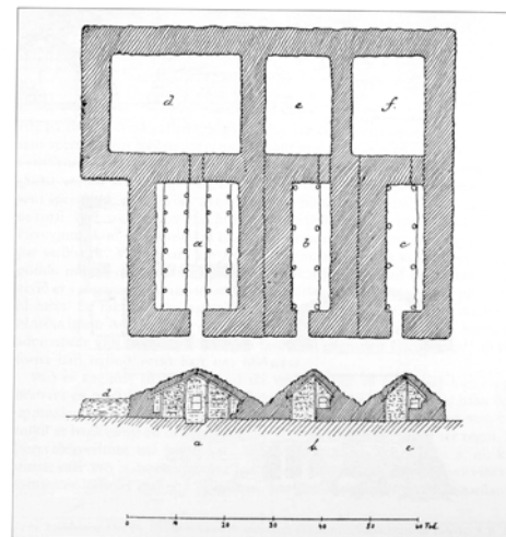
Teikning af fjósi og hesthúsum árið 1898. Hesthúsum var breytt í fjánhús og þannig notuð undir það síðasta, sjá nr. 7.
