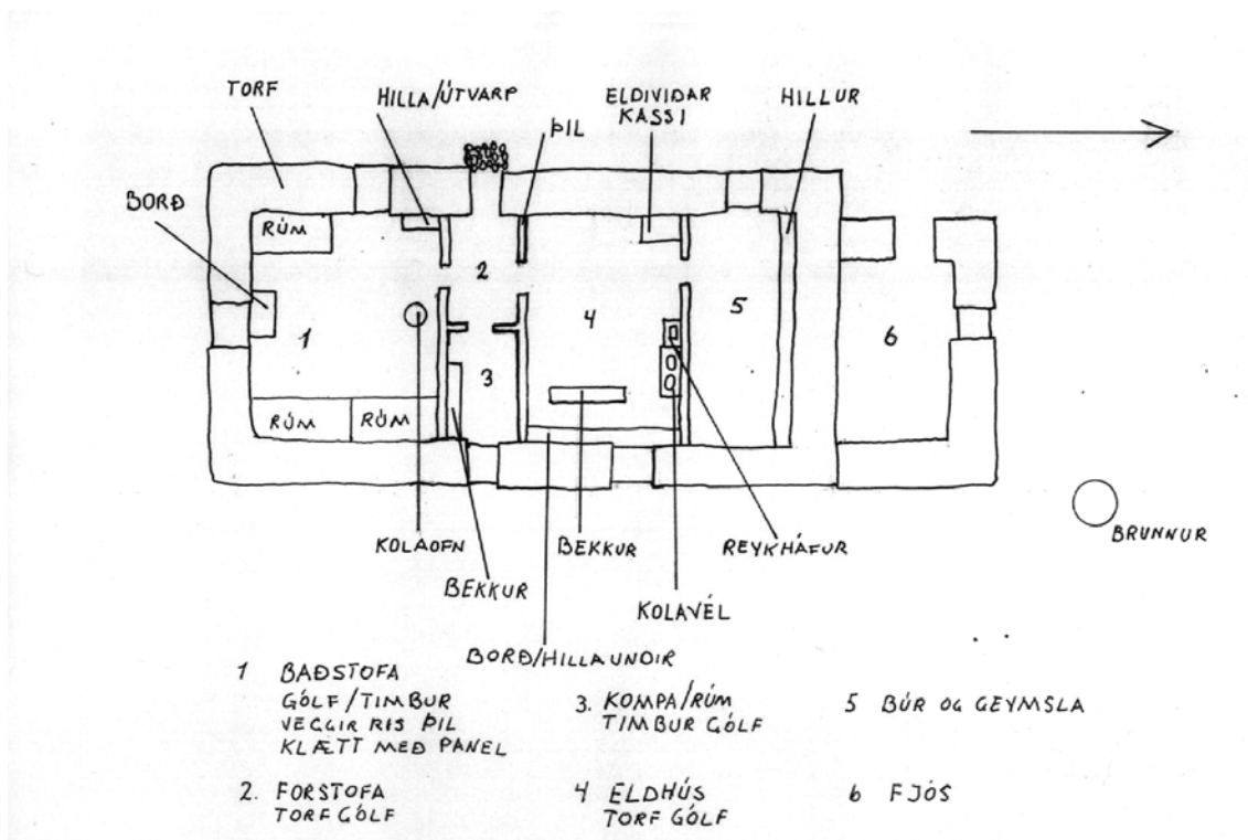
Mynd 58. Flatarteikning af Þangstaðabænum gerð eftir frásögn Jakobs Einarssonar í október 2000. Teikn. K.G. 2000.
