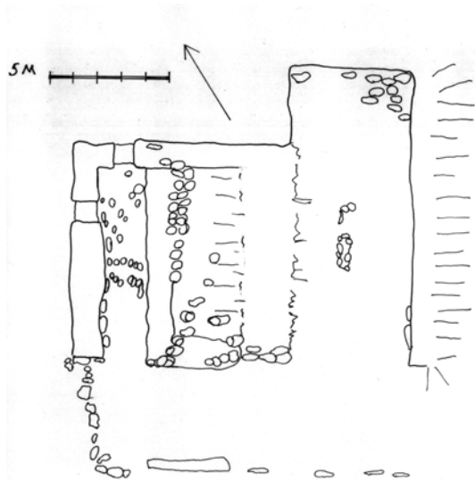
Mynd 12. Flatarteikning, hleðsla nr. 9, Teikn. K.G. sept. 2000
