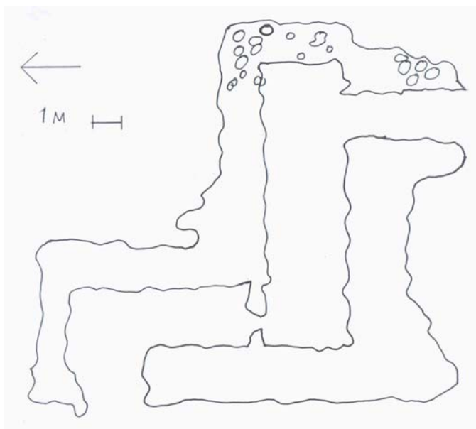
Mynd 10. Flatarteiknin, fjárhús tóft. Teikn. K.G. 1999
