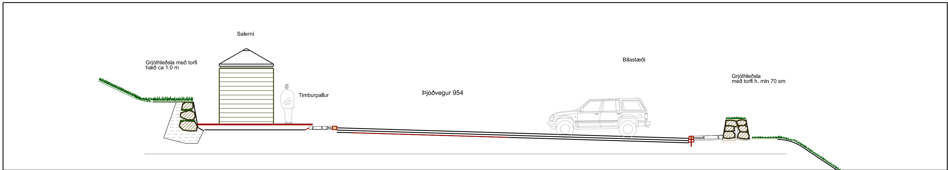
Skýringarmynd, þjónustuaðstaða Dæmisnið Mk: 1:100
