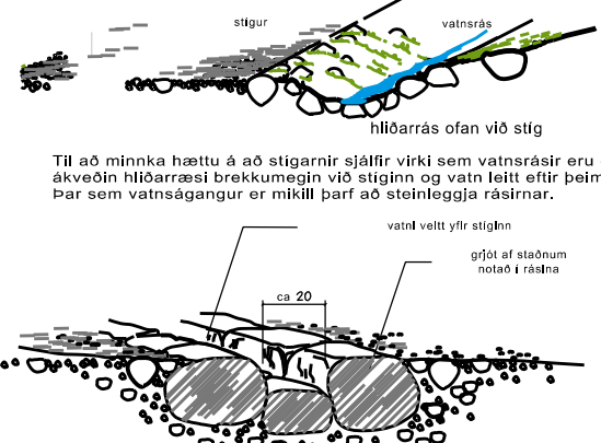
Skýringarmynd - Dæmi um frágang við stíg
