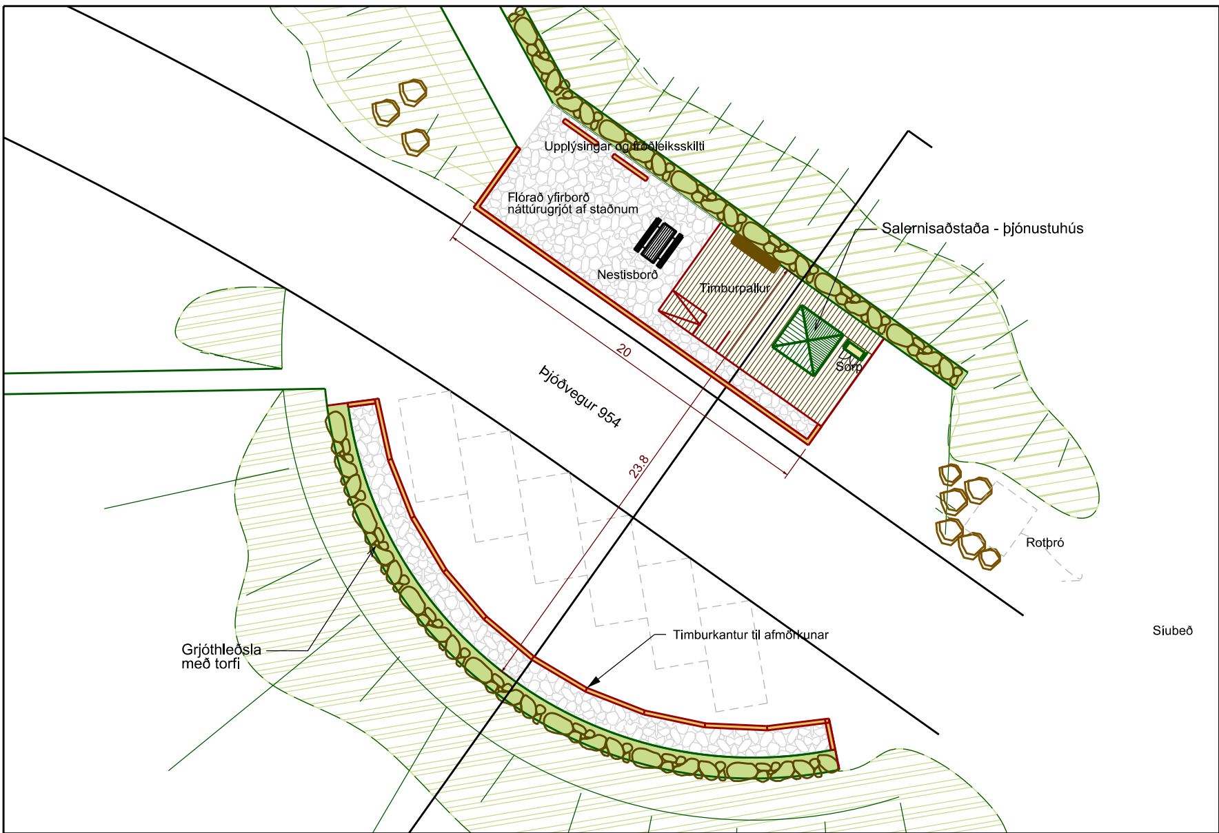
Skýringarmynd af þjónustuaðstöðu. Grunnmynd Mk: 1:250
