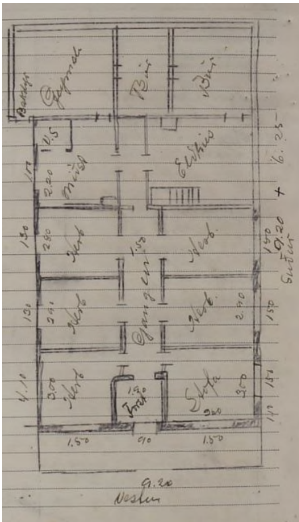
Mynd 24. Uppdráttur af íbúðarhúsinu og því sem eftir stóð af gamla bænum frá 1945 (IS HSk N00120-14-13).
