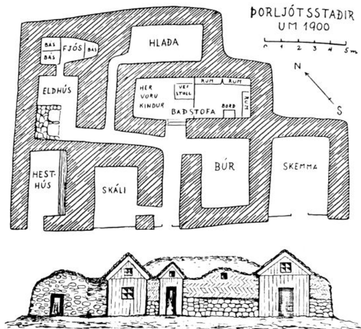
Mynd 119. Uppdráttur Kristjáns Eldjárns af bænum á Þorljótsstöðum eins og hann var um aldamótin 1900. Uppdrátturinn er birtur í bók Kristjáns Stakir steinar, 1959, bls.40. Í myndatexta segir að uppdrátturinn sé gerður eftir uppmælingum frá 1948 og eftir frásögn og teikningu Þormóðar Sveinssonar. Einnig er tekið fram að bænum hafi síðar verið breytt og hafi baðstofan verið lengd til suðurs, hlöðugangur tekinn og útidyr gerðar á fjósið.
