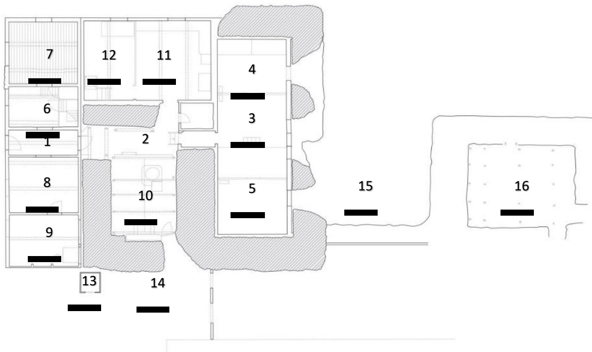
Mynd 126. Uppdráttur Hjörleifs Stefánssonar arkitekts af Vallarbænum 1999. Uppdrátturinn er einnig birtur í bók Hjörleifs Af jörðu, bls. 145. 1. bæjardyr, 2. göng, 3. miðbaðstofa, 4. suðurhús, 5. norðurhús, 6. símakompa og stigi upp á loft, 7. sparistofa, 8. norðurstofa, 9. norðurskemma, 10. hlóðeldhús, 11. eldhús, 12. búr og þar stigi upp á loft, 13. kamar, 14. rústir brunnhúss, 15. rétt, 16. fjósið og síðar hrútakofi.
