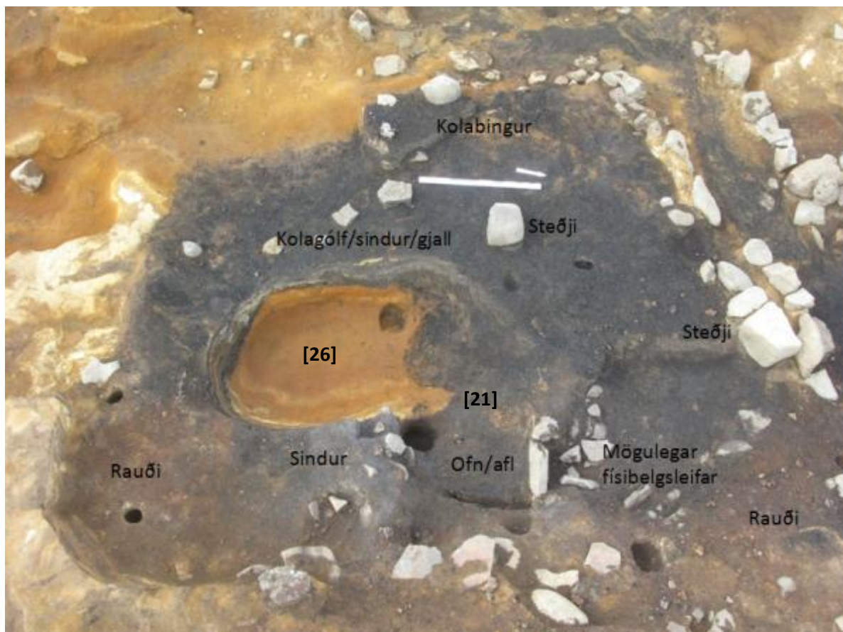
Mynd 44. Mynd af gólfi í rauðasmiðju A7 sem er eldri smiðjan af tveimur frá því fljótlega eftir 940 og einhvern tíma fyrir 1104. Norðurör og 1m skali eru ofarlega fyrir miðri mynd, milli kolabings (sem var að vísu yngri en gólfið) og steinsteðja. Búið er að hreinsa uppúr niðurgreftri [26] fyrir miðju hússins, en hann var hluti af raski frá A5. Syðst í niðurgreftrinum var lítill afl [29] settur saman úr fjórum gjallkökum. Hægra megin við efri steðjasteinin kom í ljós botn annars bræðsluofns [22] þegar gólfið var lækkað. Ofn [21] er neðarlega fyrir miðri mynd.
