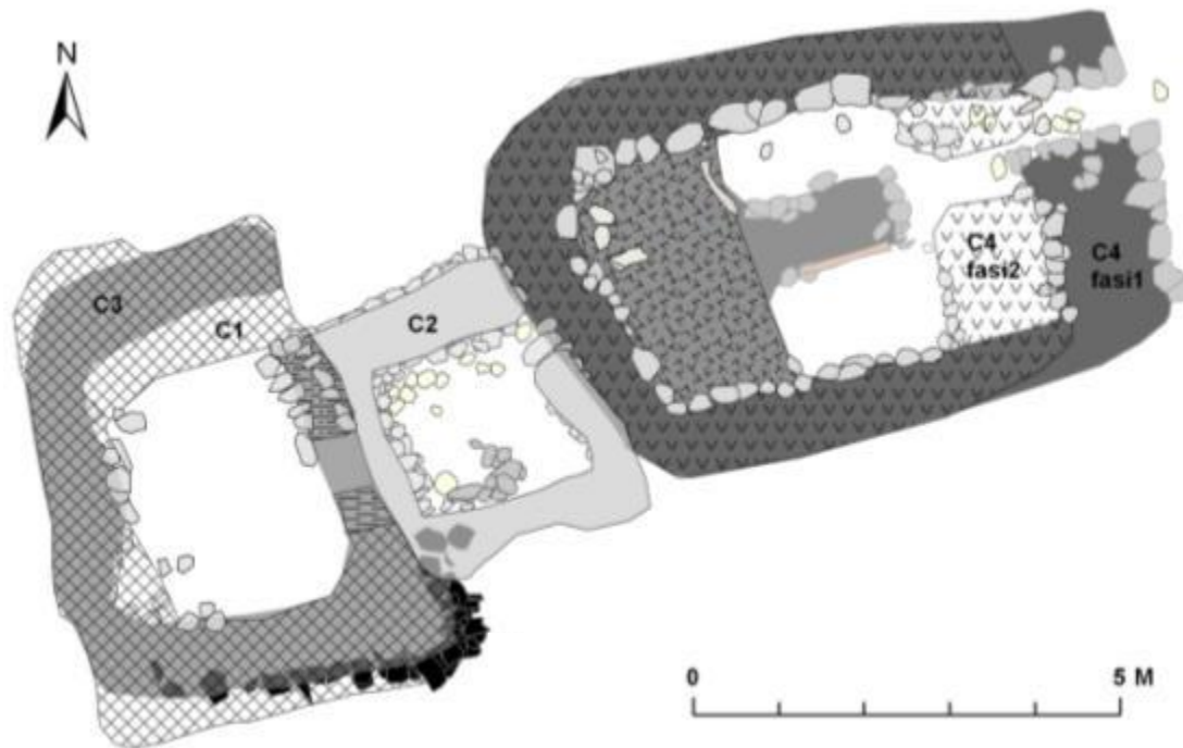
Mynd 79. Yfirlitstekning af byggingum á svæði C. Torf sem talið var tilheyra C3 hafði fallið inn í tóftin að sunnan og austan og voru eiginlegar innbrúnir byggingarinnar við svörtu steinana sem sýndir eru á myndinni.
