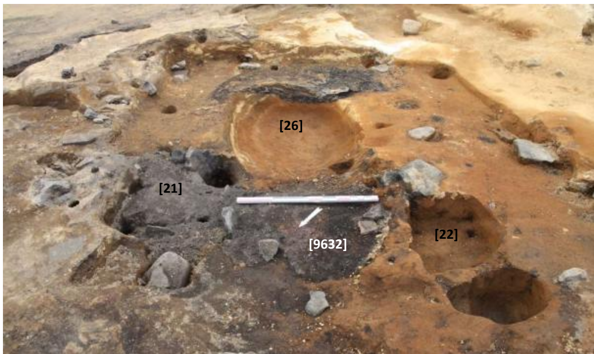
Mynd 49. Horft til suðvesturs yfir rauðasmiðju A7, búið er að fjarlægja gólfið [3619] að mestu, sem og hreinsa uppúr vestari bræðsluofninum [22]. Sjá má stoðarholur og –steina meðfram útveggjum og hægra megin við niðurgröftinn í miðjunni [26]. Fig. 49. Looking southwest over smelting hut A7. The floor [3619] almost fully excavated, as well as the west furnace [22]. Post stones and post holes can be seen along the outer walls and to the right of the truncation in the middle of the building.
