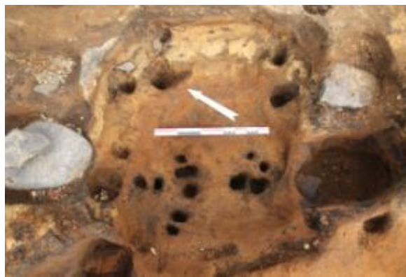
Mynd 48. Botn í ofni [21]. Fig. 48. Bottom of furnace [21].
