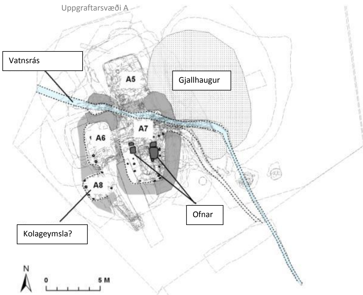
Mynd 41. Eldri rauðasmiðja A7 og járnvinnslusvæðið fyrir 1104.
