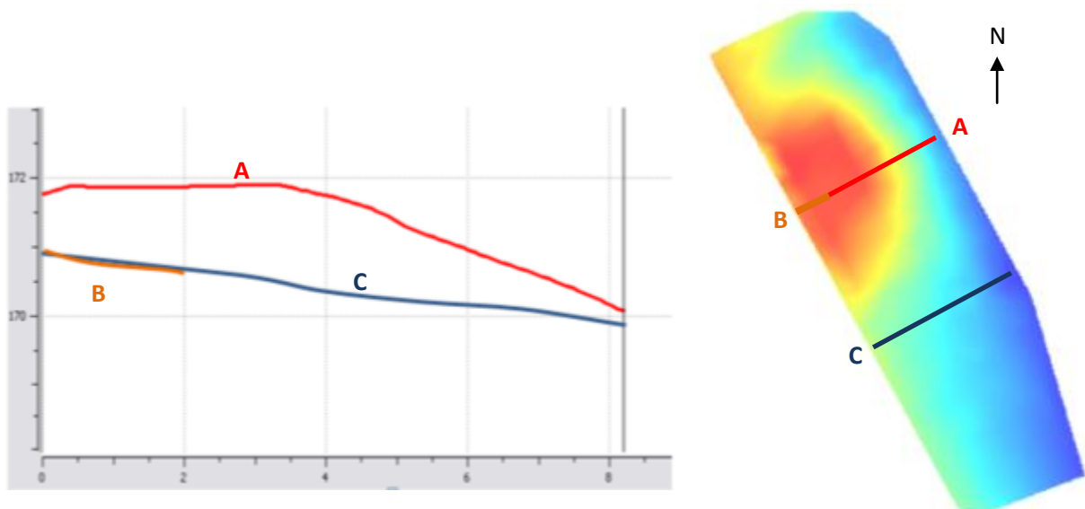
Mynd 76. Snið í gegnum gjallhaug, beint út frá inngangi inn í yngri rauðasmiðjuna. Lóðrétti ásinn sýnir raunhæð yfir sjávarmáli og lárétti ásinn metra út frá veggjum smiðjunnar til NA. Þunnt lag af sótugu efni og smáræði af gjalli teygði sig lengra til norðausturs, alls rúma 9m frá veggjum A5. Lína A er yfirborð gjallhaugsins, lína B er botninn undir vestanverðum gjallhaugnum. Lína C er hæðarlína tekinn rétt sunnan við gjallhauginn til samanburðar.
