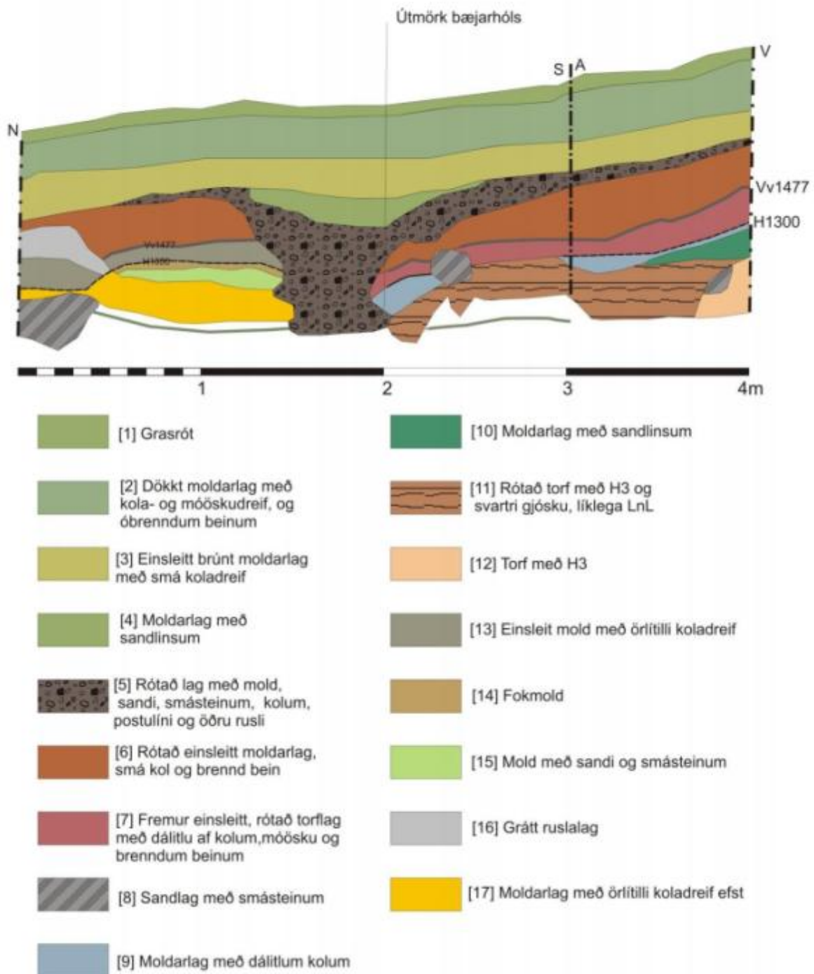
Mynd 101. Sniðteikning úr skurði 11-'11 (Guðný Zoëga 2011. Bls. 25).
