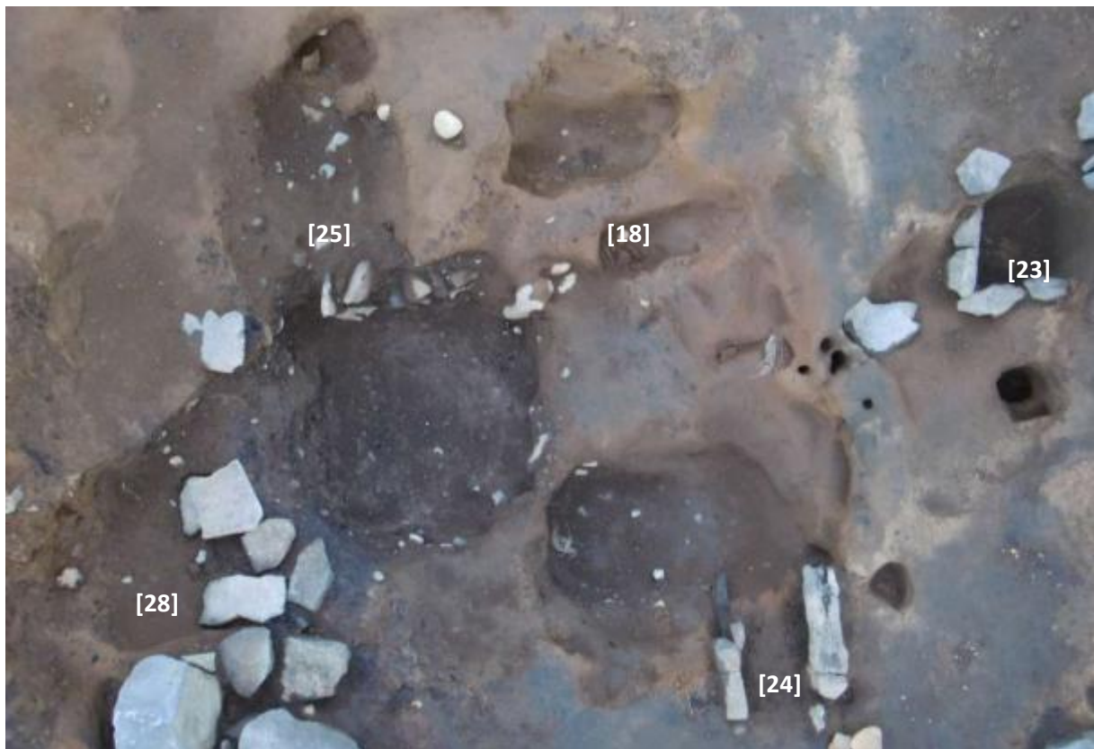
Mynd 30. Leifar ofna og afla í yngri rauðasmiðjunni A5. Leifar ofns [25] höfðu þegar myndin var tekin orðið fyrir smávægilegu raski þar sem haftið milli ofnsins og holunnar norðan við hafði hrunið.
