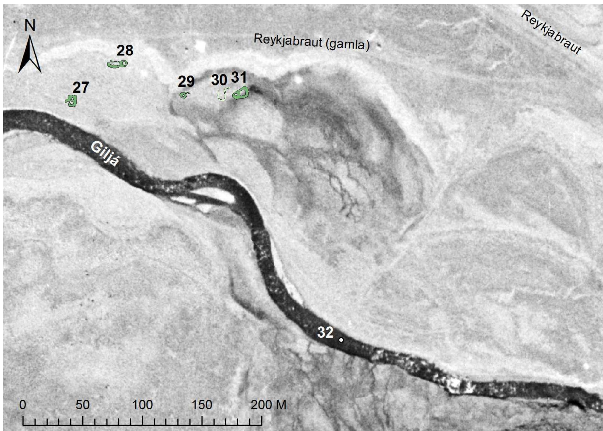
Mynd 9, minjar í Norðlingahvammi við Giljá. Loftmynd Landmælingar Íslands (M14-M-2986).
