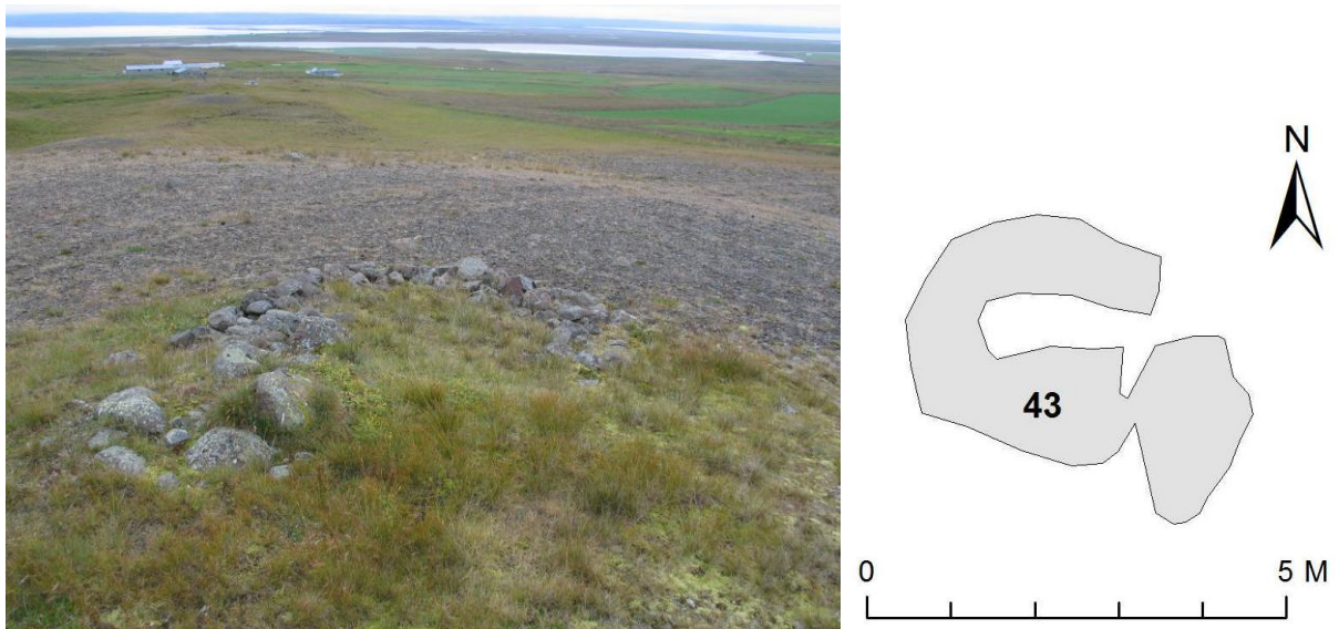
Mynd 17, horft til vesturs yfir steinklögn (nr. 43) austur af Beinakeldu, í baksýn er útihúsin á Beinakeldu og rétt glittir í þakið á íbúðarhúsinu.
