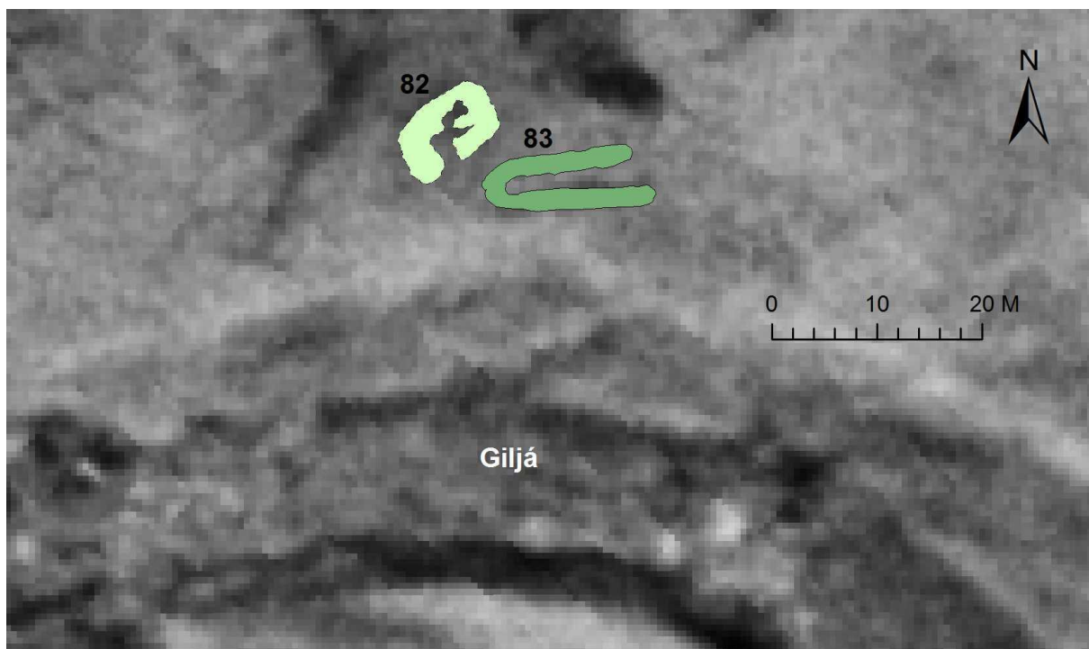
Mynd 32, minjar við Giljá þar sem hún sveigir til vesturs fyrir mynni Sauðadals. Hugsanlega kvíar (nr. 83) og sel (nr. 82). Loftmynd Landmælingar Íslands (M14-M-2986).
