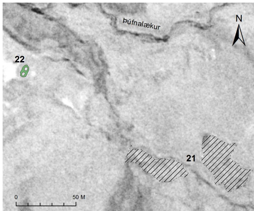
Mynd 4, mógrafir (nr. 21) í Mómýri og líklega leifar mókofa (nr. 22). Loftmynd Landmælingar Íslands (M14-M-2986).
