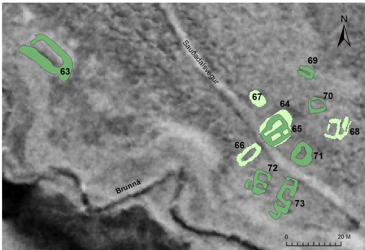
Mynd 25, minjar við Brunná, svonefndar Geirstóftir. Alls eru sjö tóftir í þyrpingu við veginn, þar af ein (nr. 65) sem virðist standa á eldra minjum (nr. 64) og ein óljós þúst (nr. 67) að auki sem kann að vísa á byggingu. Þá er stök tóft um 60m vestar í gilinu við Brunná (nr. 63). Loftmynd frá Landmælingum Íslands (M14-M-2986).
