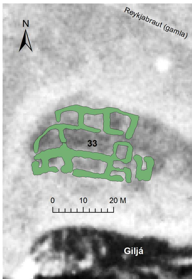
Mynd 10 rétt (nr. 33) í Réttarhvammi við Giljá. Loftmynd Landmælingar Íslands (M14-M-2986).
