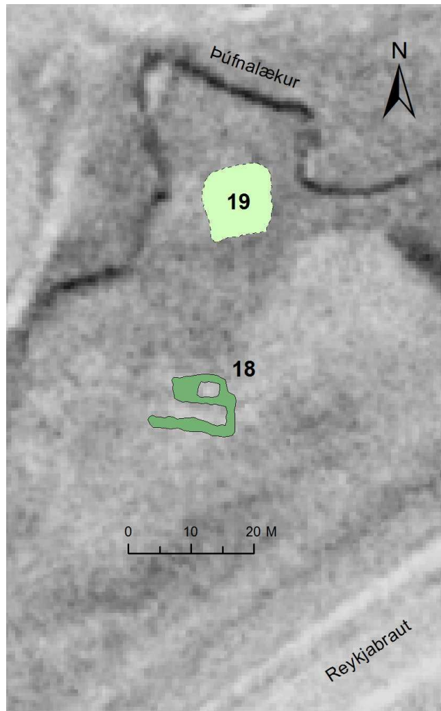
Mynd 3, þúst og stekkjartóft í Þúfnalækjargili. Loftmynd Landmælingar Íslands (M14-M-2986)
